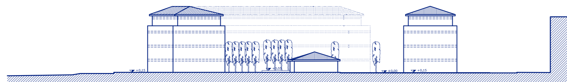
sezione C-C'
